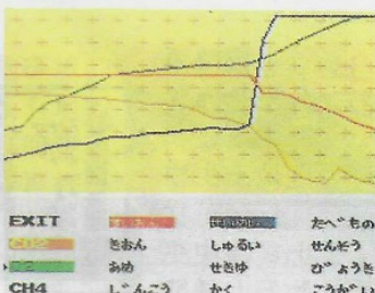
↓水蒸氣冷卻後形成海洋。生命之源就此誕生！
